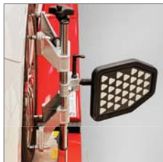
고정밀 호크아이 최신행 얼라인먼트 타겟
